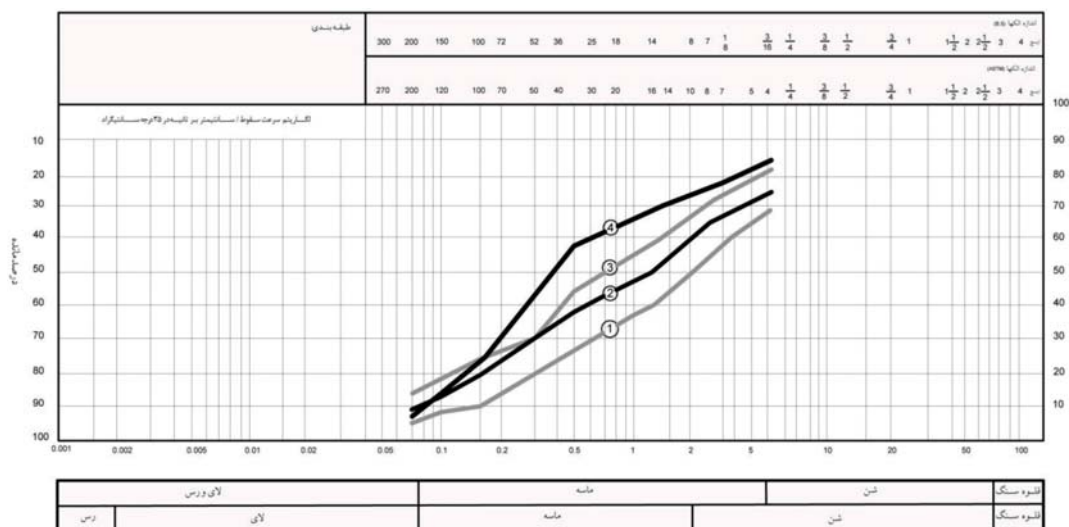
تصویر ۱. منحنی دانه بندی خاکها (۱. اصفهان، ۲. میبد، ۳. فردوس، ۴. یزد)
