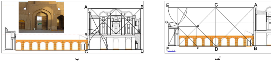
تصویر ۸. ترسیمات هندسی در مقطع (نگارندگان)
