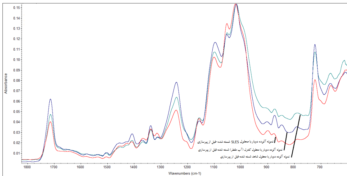
تصویر ۸. طیف ATR-FTIR پارچه آلوده دوبار شسته‌شده با محلول‌های SLES، شاهد و کنترل قبل از پیرسازی در محدوده 1800-650\text{ cm}^{-1} (نگارندگان)
