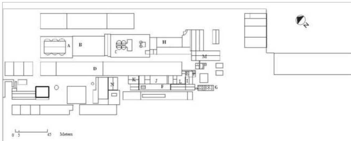
تصویر ۲. طرح فضاهای کارخانه سیمان ری؛ A و C: سیلوی سیمان، B: سالن آسیاب سیمان، D: انبار کلینکر، E و I: آسیاب مواد خام کوره ۱۰۰ تنی، F: آسیاب مواد خام کوره ۲۰۰ تنی، G: سیلوی مواد خام کوره ۳۰۰ تنی، H: تعمیرگاه، I: کوره چرخشی، N: مولد الکتریسیته (کنت، ۱۳۸۵)
